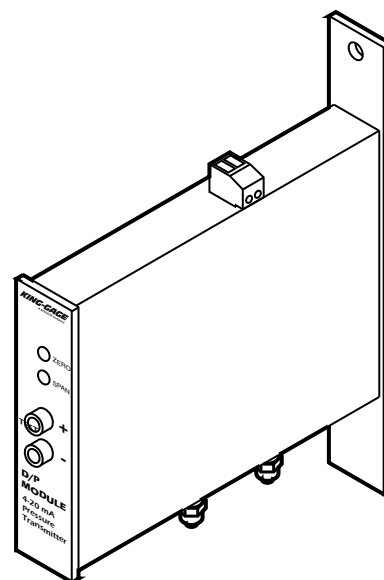
5900 D/P Module
